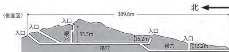
地下壕の断面図
